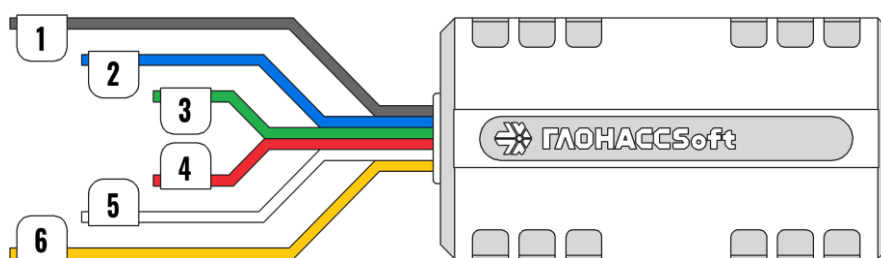
Рисунок 2.4 Нумерация выводов УМКа310
