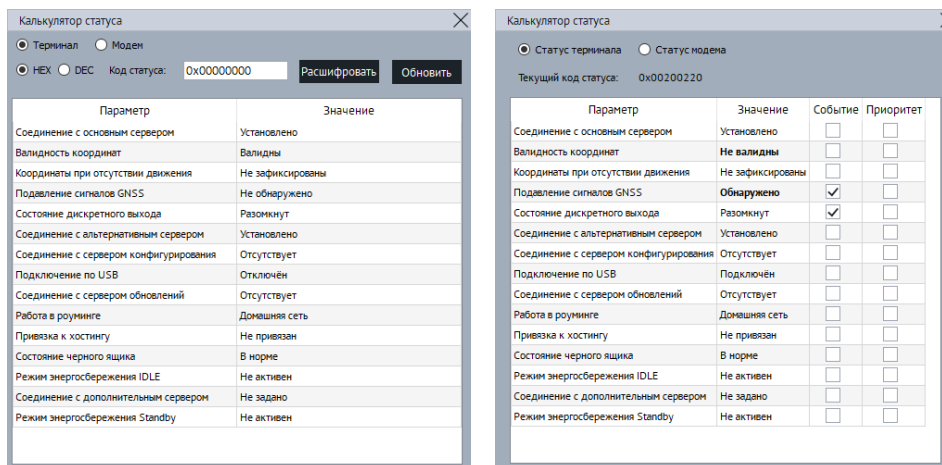
Рисунок 3.15 Калькулятор статуса
