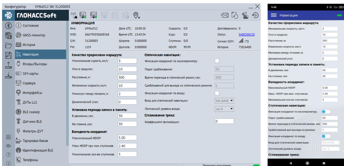
Рисунок 3.18 Вкладка «Навигация»
