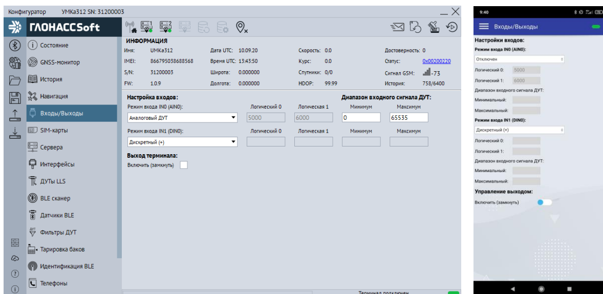
Рисунок 3.20 Вкладка «Входы/Выходы»
