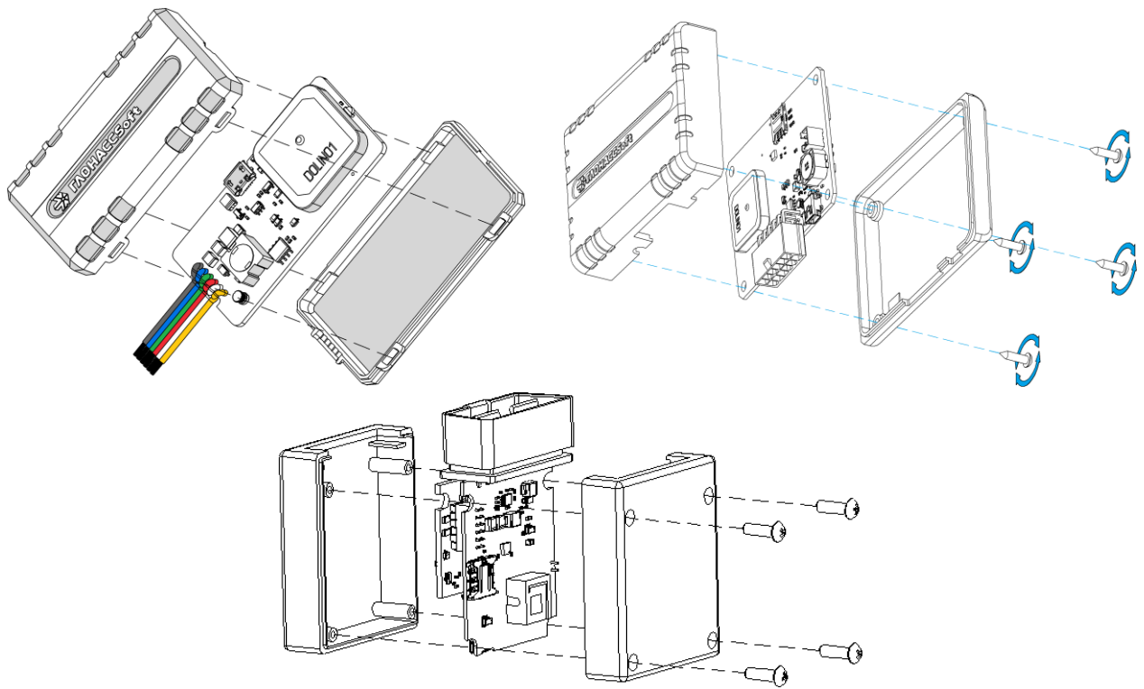
Рисунок 2.7 Вскрытие корпуса терминала (310 – слева; 312 – справа; 311 -снизу)
