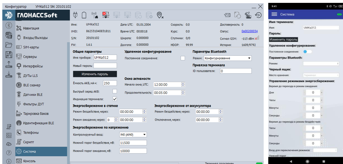
Рисунок 3.33 Вкладка «Система»
